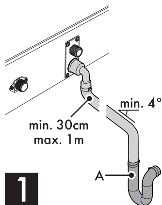
1 Непосредственный слив в канализацию
