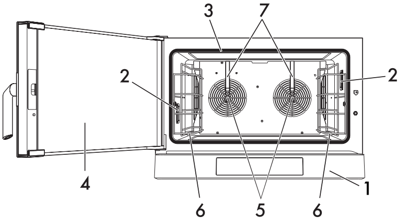
Маятниковая дверка
