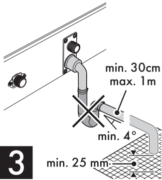
Слив через отводной коллектор
