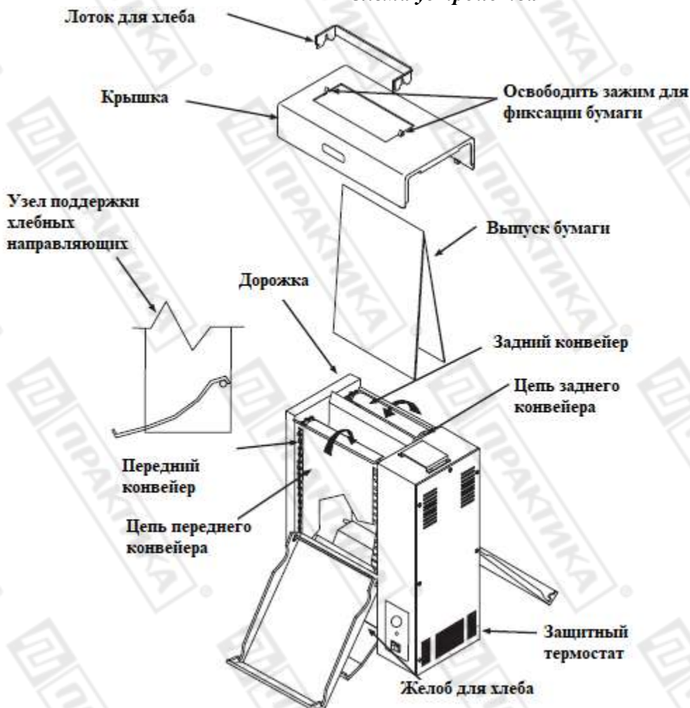
Схема устройства
